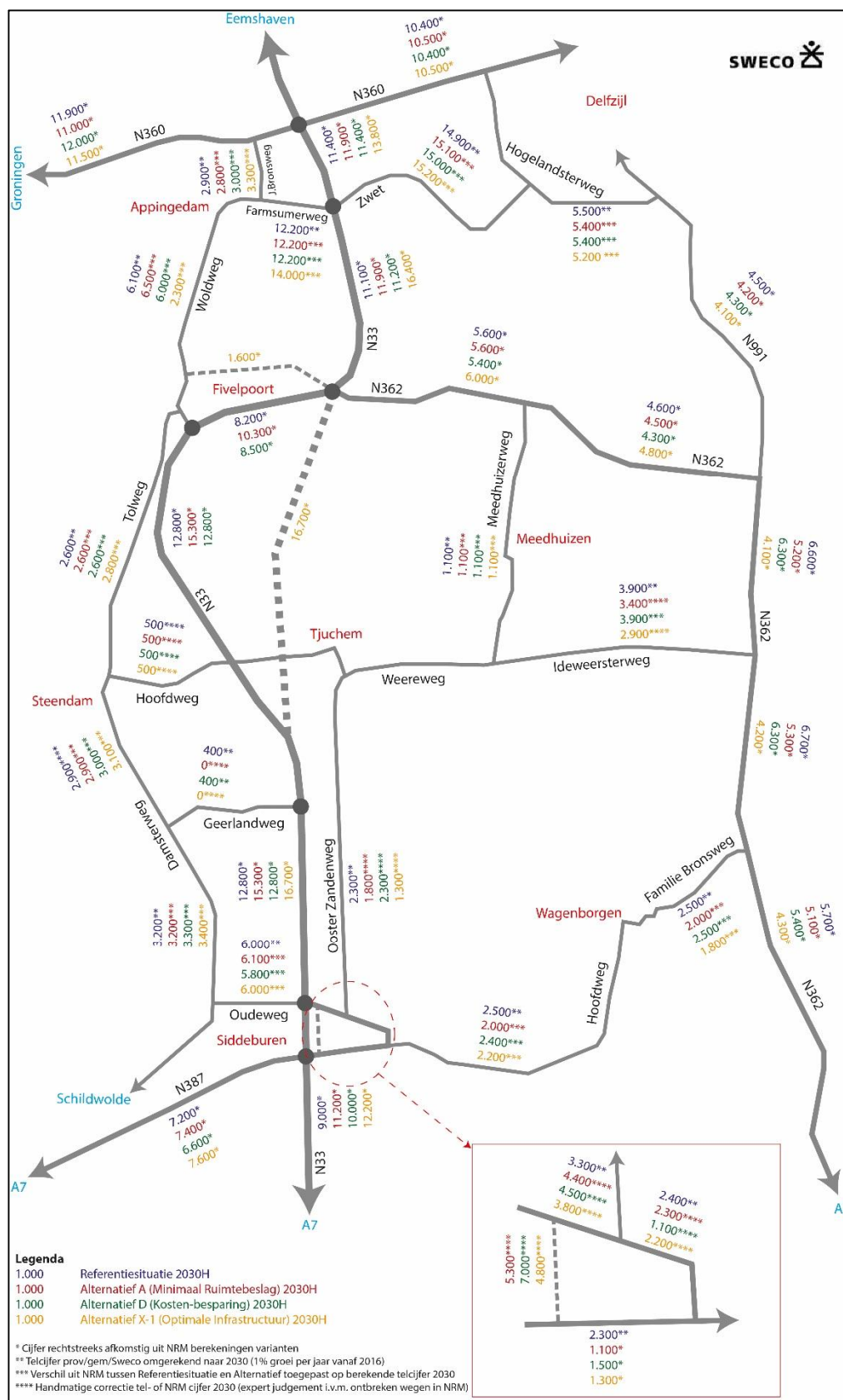
Figuur 7.2: verkeersintensiteiten hoofwegennet en onderliggend wegennet
